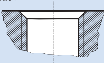
Chanfrein nécessaire conformément à DIN 76
