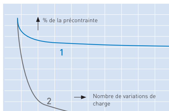
Précontrainte en cas de contrainte durable (représentation schématique)
