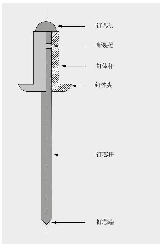
盲铆钉和断茎定义
