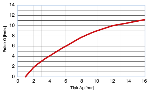
CHECK VALVE® Křivky průtoku – unscreened BF660080024100; T = 50 °C, hydraulický olej HLP46
