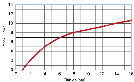
CHECK VALVE® Křivky průtoku – screened BR660080024100; T = 50 °C, hydraulický olej HLP46
