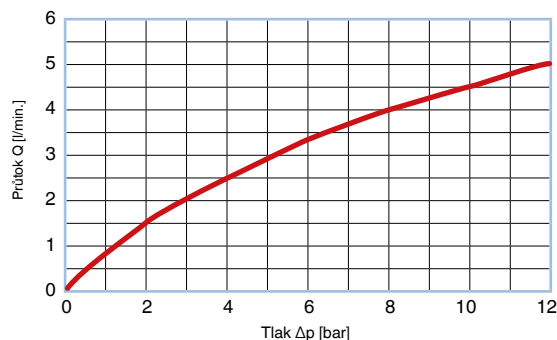
CHECK VALVE® Křivky průtoku – unscreened BFAA055U014; T = 50 °C, hydraulický olej HLP46
