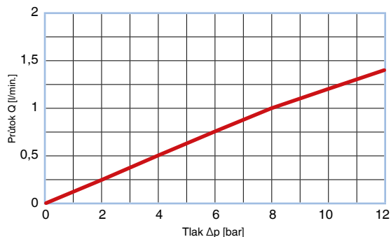
CHECK VALVE® Křivky průtoku – screened BFAA055014; T = 50 °C, hydraulický olej HLP46
