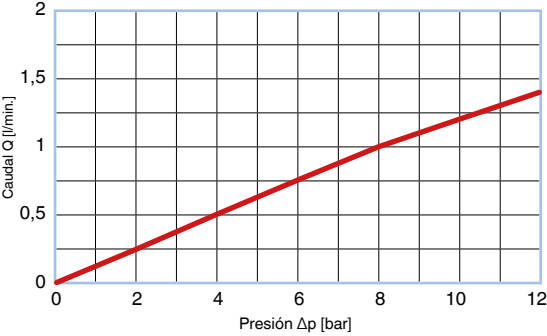
Curva caudal-presión, CHECK VALVE® – con tamiz BFAA055014; T = 50 °C, Aceite hidráulico HLP46
