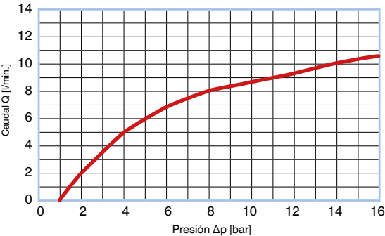
Curva caudal-presión, CHECK VALVE® – con tamiz BR660080024100; T = 50 °C, Aceite hidráulico HLP46
