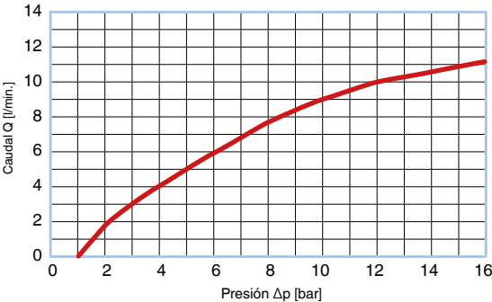
Curva caudal-presión, CHECK VALVE® – sin tamiz BF660080024100; T = 50 °C, Aceite hidráulico HLP46
