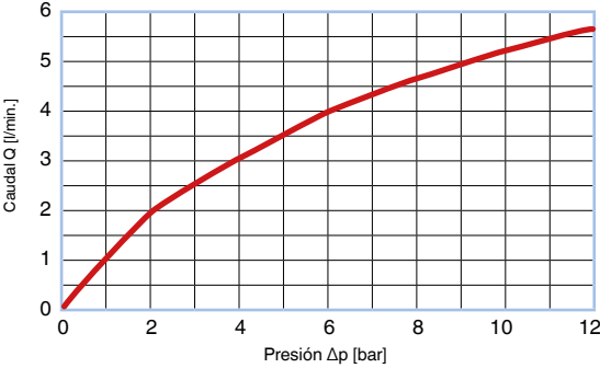
Curva caudal-presión, CHECK VALVE® – sin tamiz BFAA055U014; T = 50 °C, Aceite hidráulico HLP46
