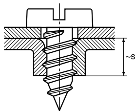
4. agujero para roscar punzonado y extrudido (láminas finas)
