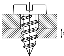
2. atornillamiento simple (con agujero pasante)
