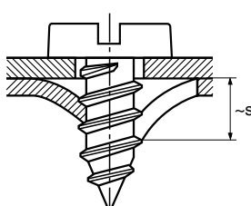
5. atornillamiento de agujero de presión
