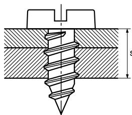
1. atornillamiento simple (dos agujeros para roscar)
