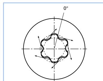
0° de ángulo de aplicación de la fuerza en el accionamiento Torx plus®
