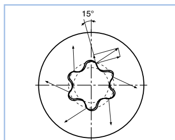
15° de ángulo de aplicación de la fuerza en el accionamiento de accionamiento hexalobular interior
