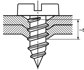
3. agujero para roscar mandrilado (láminas finas)
