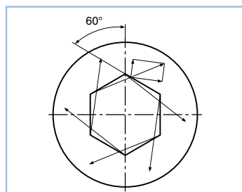
60° de ángulo de aplicación de la fuerza en el accionamiento de hexágono interior
