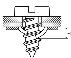
6. atornillamiento con tuerca de resorte de apriete
