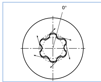
0° Kraftangrebsvinkel ved Torx plus® kærven
