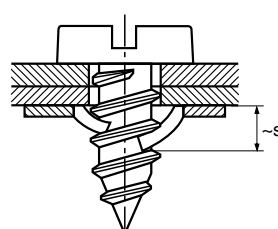
6. Skrueforbindelse med klipsmøtrik
