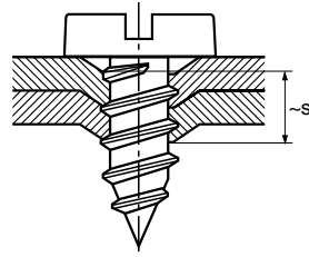
3. Kernehul opkravet (tynd plade)
