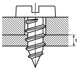
2. Enkel skruesamling (med gennemgangshul)
