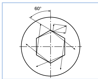
60° Kraftangrebsvinkel ved indvendig sekskant
