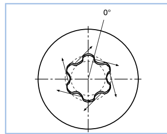
Úhel přenosu síly 0° u Torx plus®
