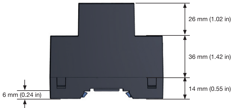
Vista izquierda
