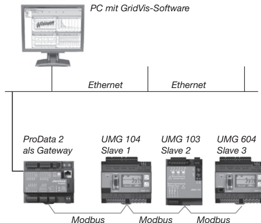
Abb.: Anschlussvariante mit ProData 2 als Gateway. Das Prodata 2 setzt die Anfragen der Software GridVis (TCP-Pakete über Ethernet) für die Modbus-Slavegeräte (Modbus RTU) um und leitet diese über die RS485-Schnittstelle weiter (RS485-Modus: Gateway; Adr.3=1).
